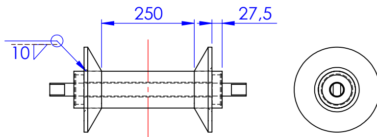
MONTAGEM DA GUIA NO ROLO
