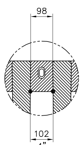
DETAIHE "Y" ESC. 1:10
