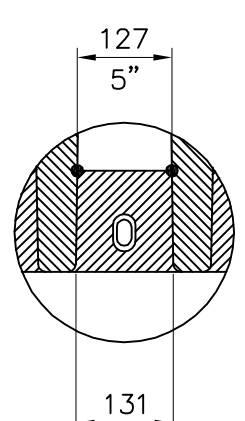
DETALHE "Z" ESC. 1:10
