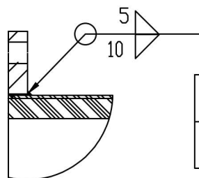
DETALHE TÍPICO FLANGE FIXO
