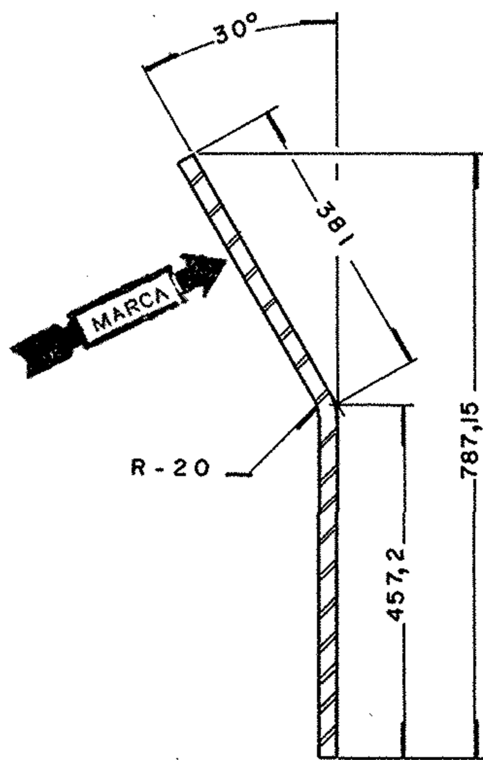
SEÇÃO "Z-Z"
