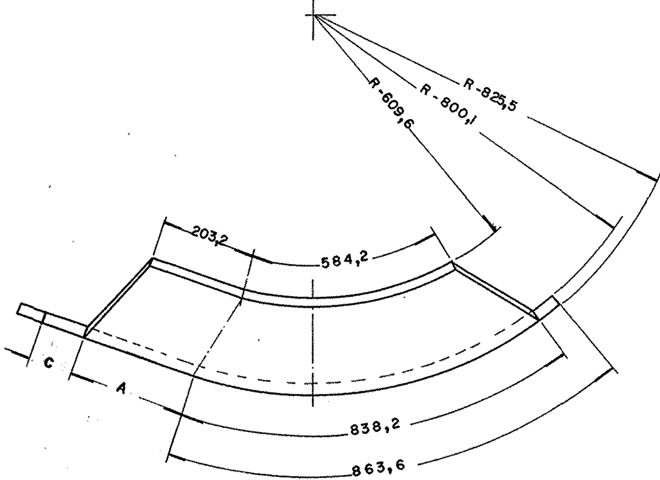
PEÇA Nº 2-3
