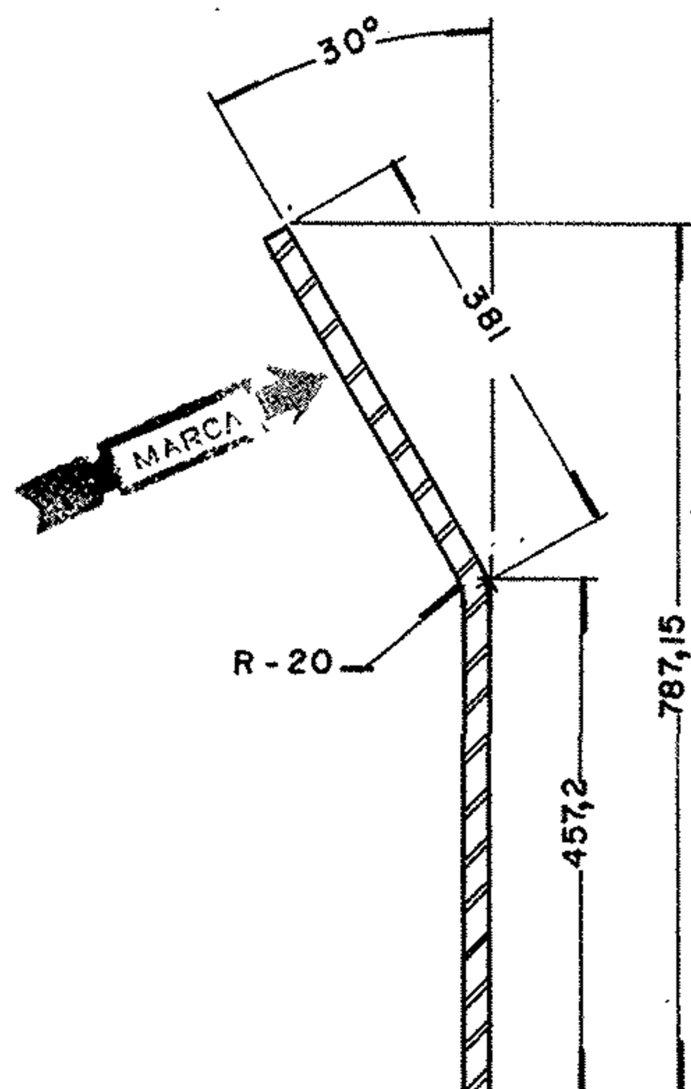
SEÇÃO "X-X"
