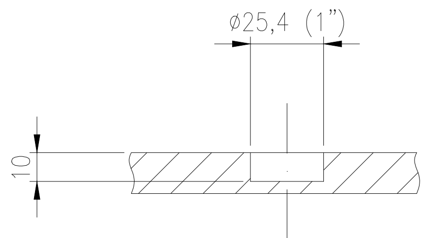
DETALHE A ESCALA 1:2,5
