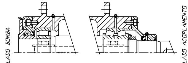
DETALHE DE MONTAGEM DOS RETENTORES
