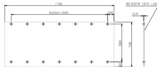
DETALHE BL07
