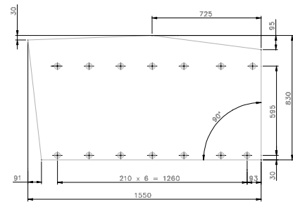
DETALHE BL13
