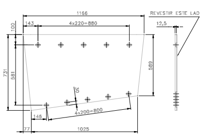
DETALHE BL11
