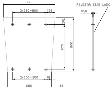
DETALHE BL05
