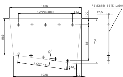
DETALHE BL02
