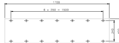
DETALHE BL15
