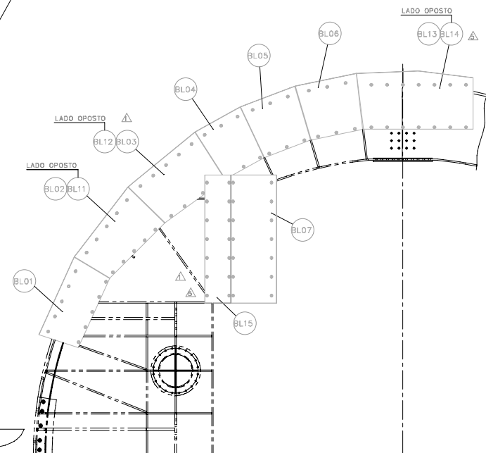
DETALHE TÍP. FIXAÇÃO DO REVESTIMENTO ESC. 1:2
