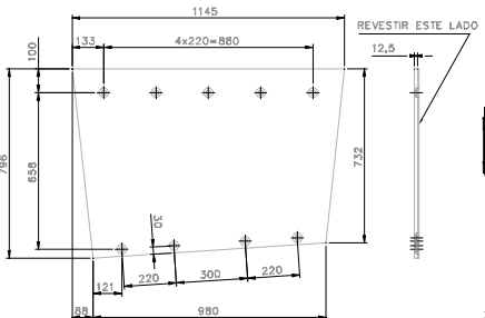
DETALHE BL12
