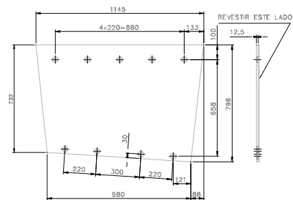
DETALHE BL03
