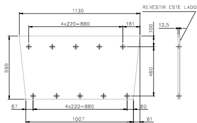
DETALHE BL01
