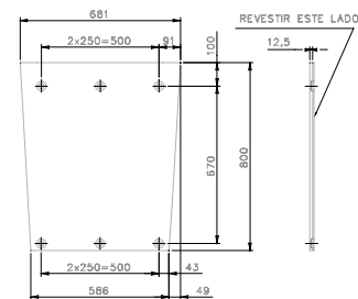
DETALHE BL04
