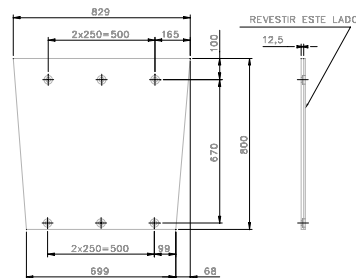
DETALHE BL06
