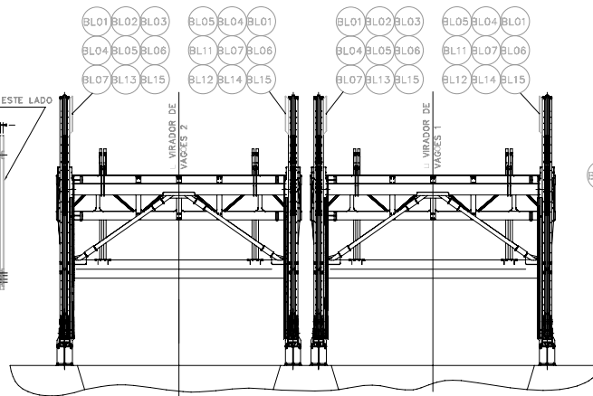
ESQUEMA DOS VIRADORES ESC. 1:100
