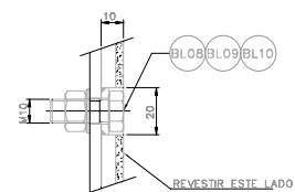
DETALHE TÍP. FIXAÇÃO DO REVESTIMENTO ESC. 1:2
