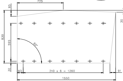
DETALHE BL14
