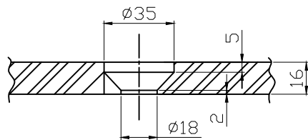
CORTE "AA" ESCALA 1:2
