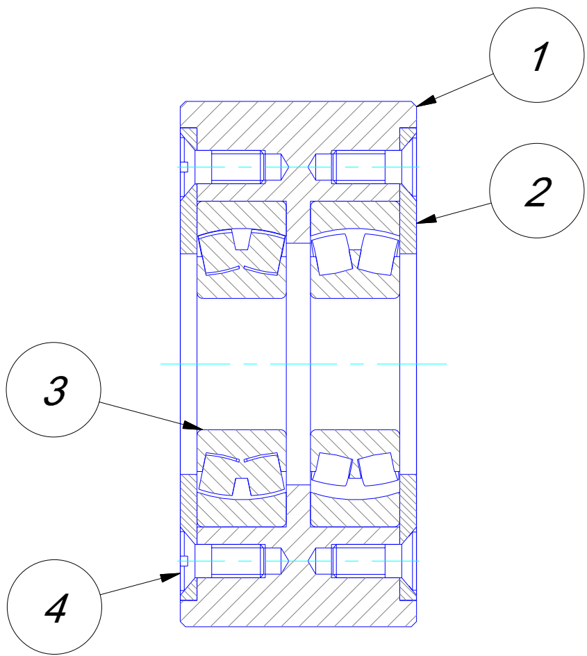
CORTE A-A (1 : 1,5)
