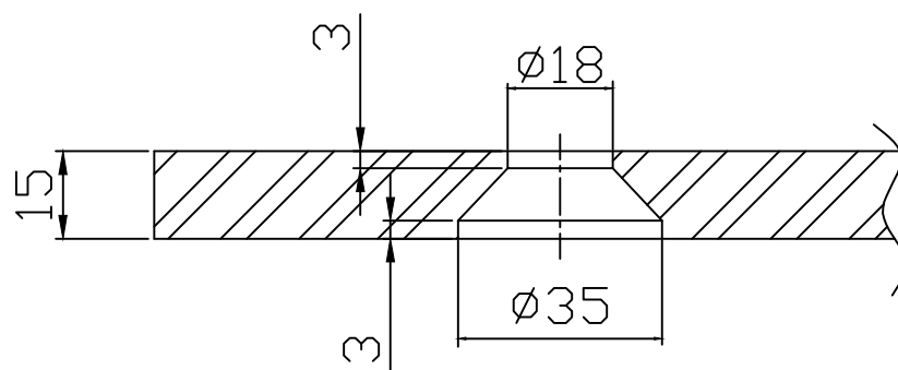
CORTE "AA" ESCALA 1:2
