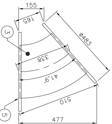
CURVA "B" - MOINHO 1 Esc: 1:10
