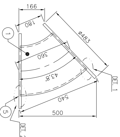
CURVA "A" – MOINHO 1 ESC.: 1:10
