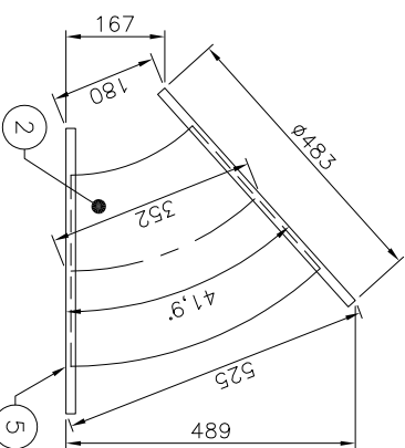
CURVA "A" – MOINHO 3 ESC: 1:10
