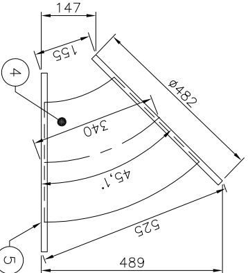
CURVA "B" – MOINHO 3 ESC: 1:10
