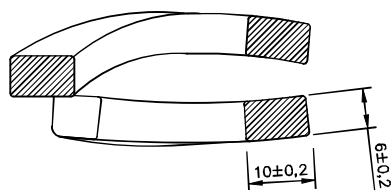
CORTE E-F
