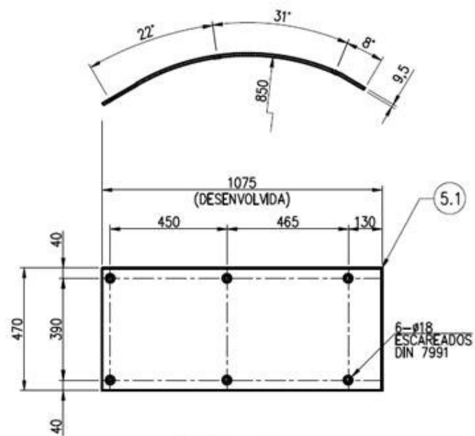
ITEM 5 ESC.: 1:15
