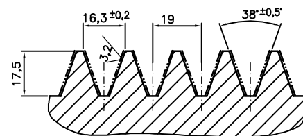
DETALHE Z
