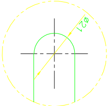
DETALHE "1" TÍP.
