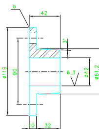
CORTE A-A
