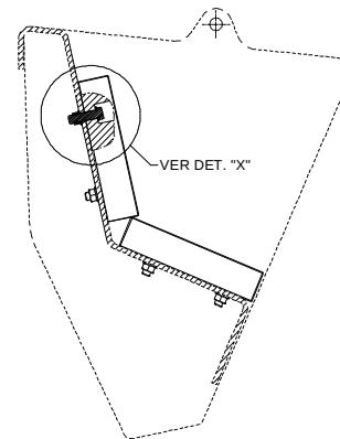
CORTE B-B ESC.: 1:7,5
