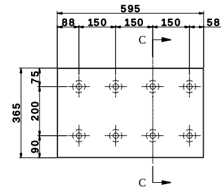
ITEM 1 ESC.: 1:7,5
