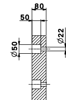
CORTE C-C ESC.: 1:7,5
