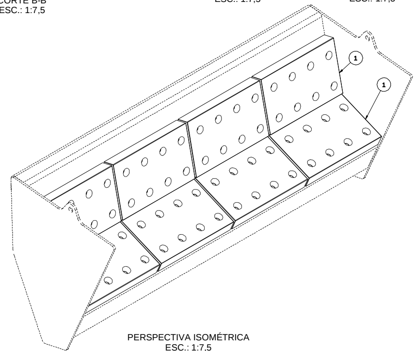
ITEM 1 ESC.: 1:7,5
