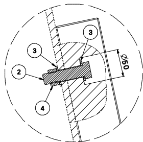
DETALHE "X" ESC.: 1:2,5
